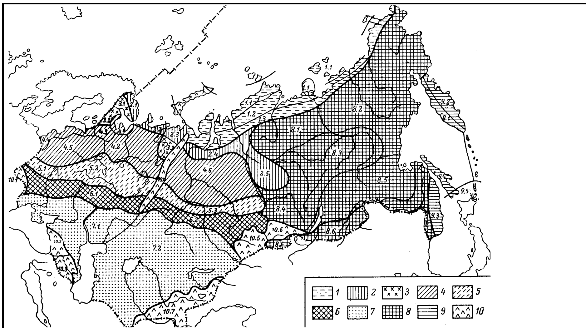
Рис. 1. Картограмма болотных зон и провинций: 1- зона полигональных болот; 2 - зона бугристых болот; 3 - группа провинций аапа-болот; 4 - зона выпуклых грядово-мочажинных болот; 5 - зона сосново-сфагновых верховых и низинных травяных болот; 6 - зона низинных осоковых и тростниковых болот; 7 - зона пресноводных и засоленных травянистых болот; 8 - континентальные провинции Сибири; 9 - приморские провинции Дальнего Востока; 10 - высокогорные провинции (по Боч, Мазинг, 1979).
